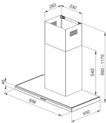
Schemi dimensionali e di installazione
