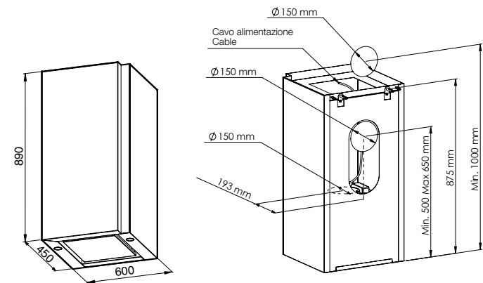
Schemi dimensionali e di installazione
