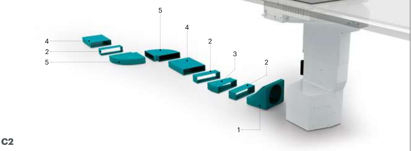
INSTALLAZIONE IN MOBILI CON ZOCCOLO H=6cm Riferimento accessori pag. 150
