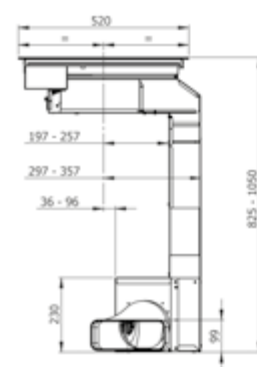
Motore frontale
