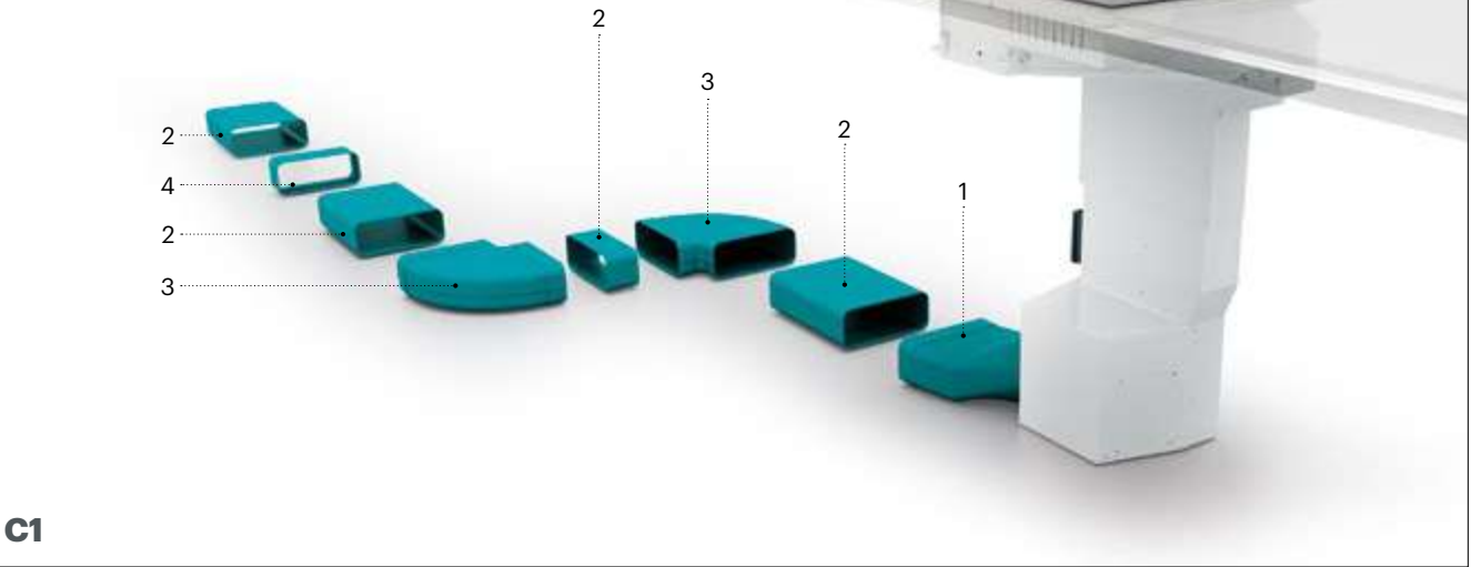
INSTALLAZIONE IN MOBILI CON ZOCCOLO H=10cm Riferimento accessori pag. 150
