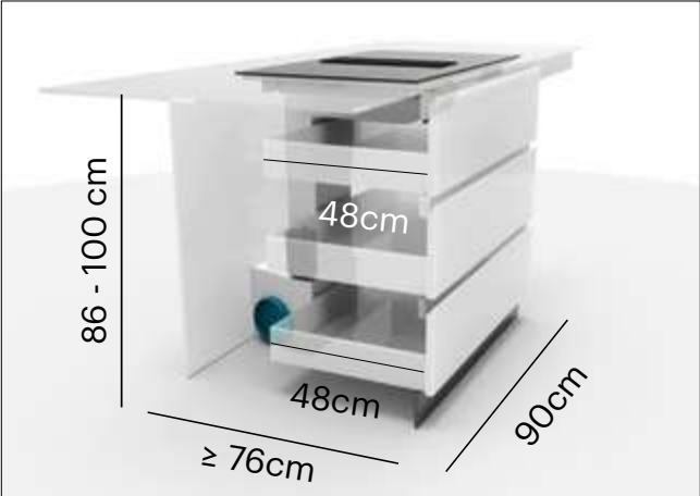
Base ≥ 76 - scarico a sinistra
