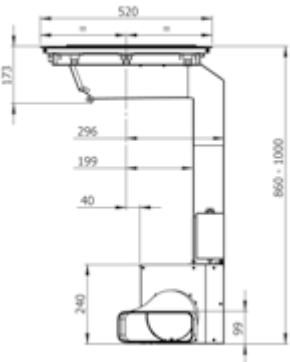
Motore frontale
