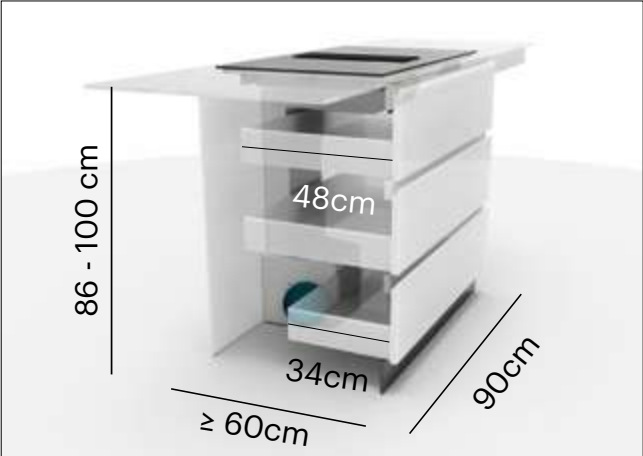
Base ≥ 60 - scarico a sinistra
