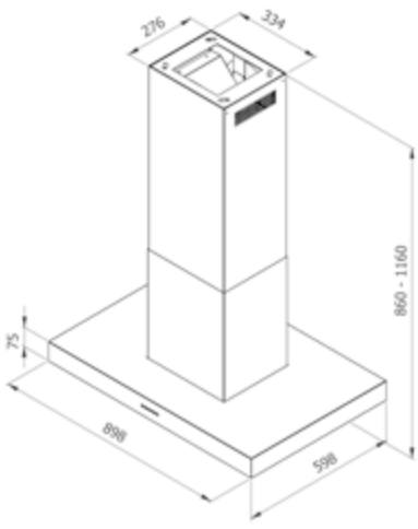
Schemi dimensionali e di installazione
